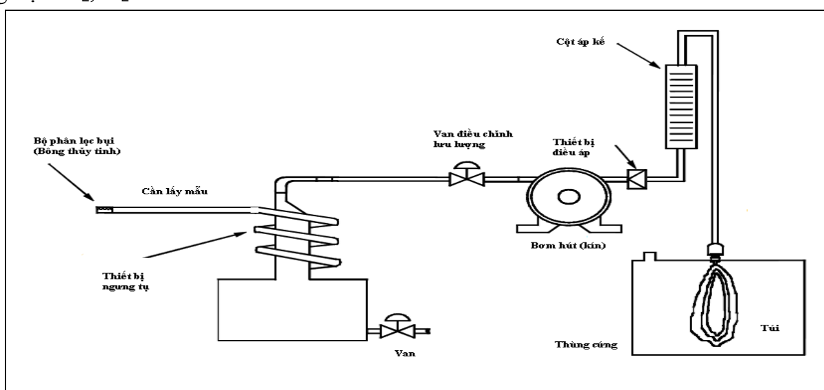
Hình 14: Bộ thu mẫu tổ hợp
