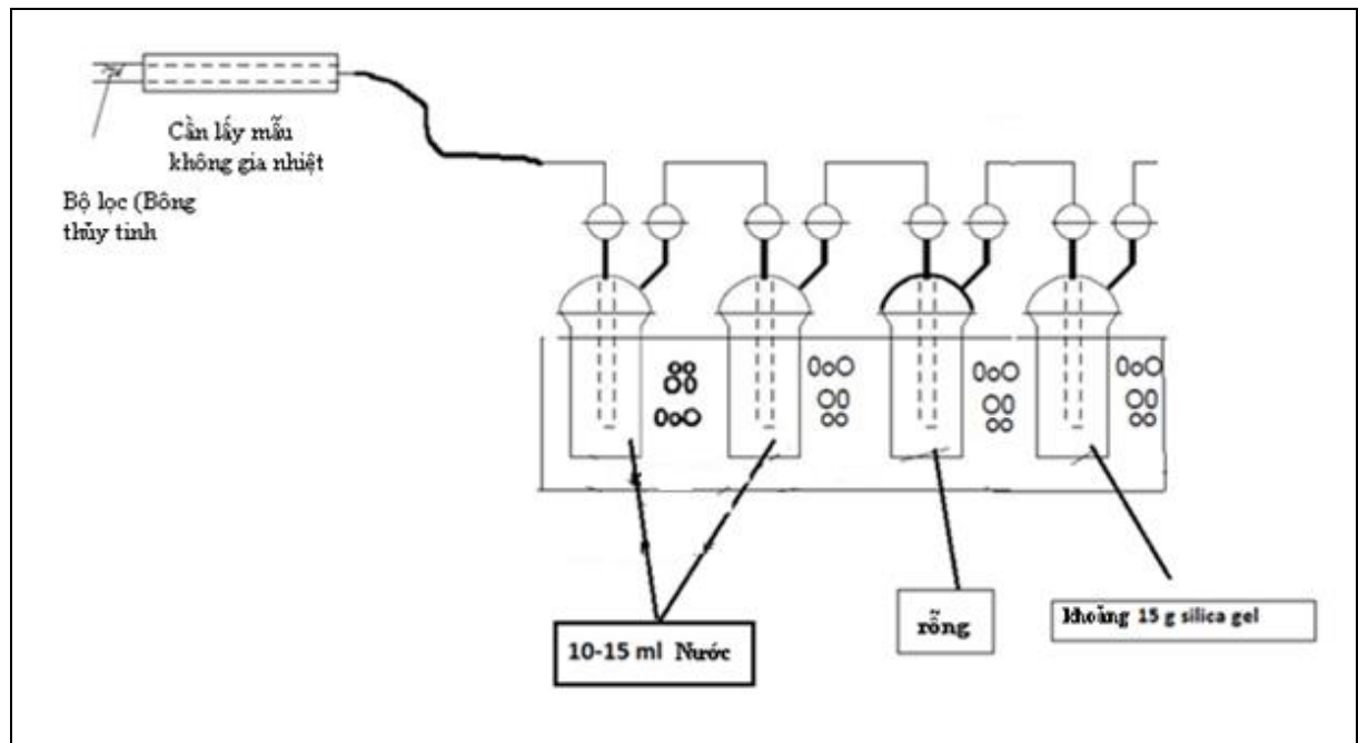
Hình 16: Hệ thống các impinger trong ống khói
